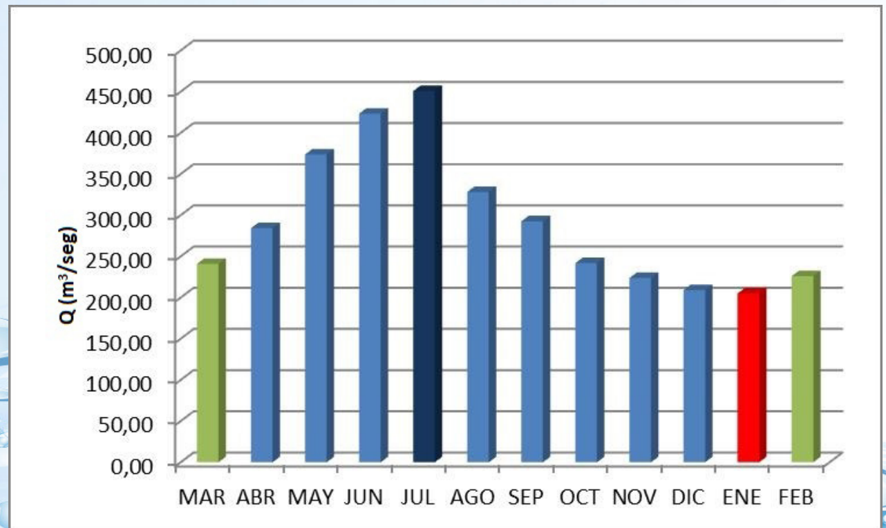
Figura 4. Régimen Hidrológico, estación hidrológica Jatunyacu DJ Illoculin (H0721). Elaborado por: Equipo Técnico Secretaría del Agua, 201
