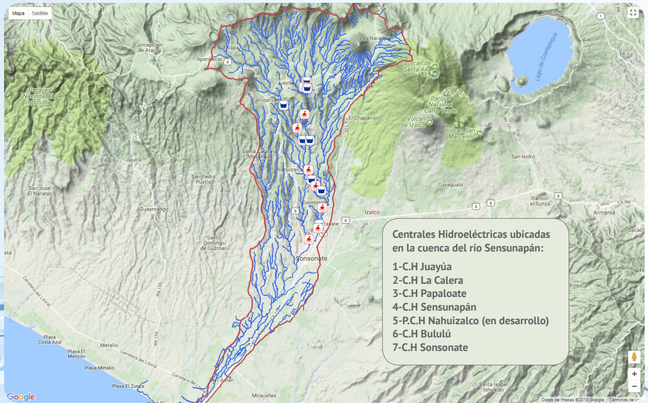
Figura 2. Ubicación de pequeñas Centrales Hidroeléctricas sobre río Sensunapán
