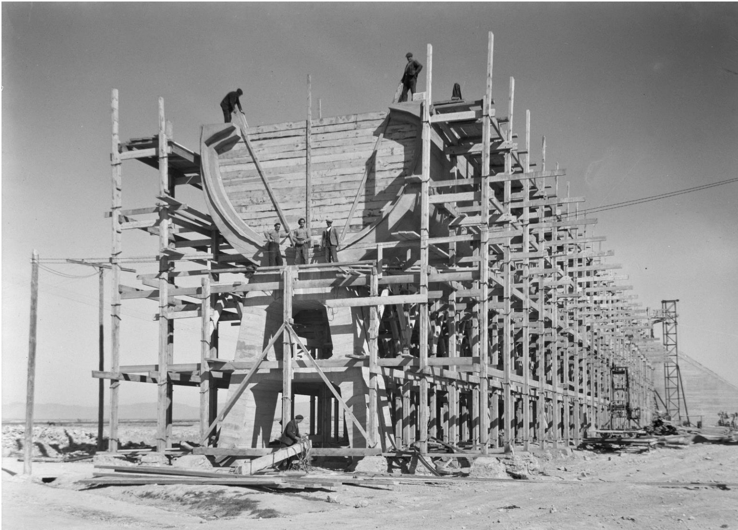
Construcción del acueducto de Tardienta, 1935
